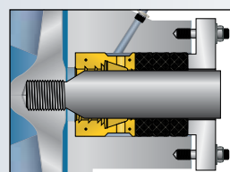
Šnúrová upchávka
